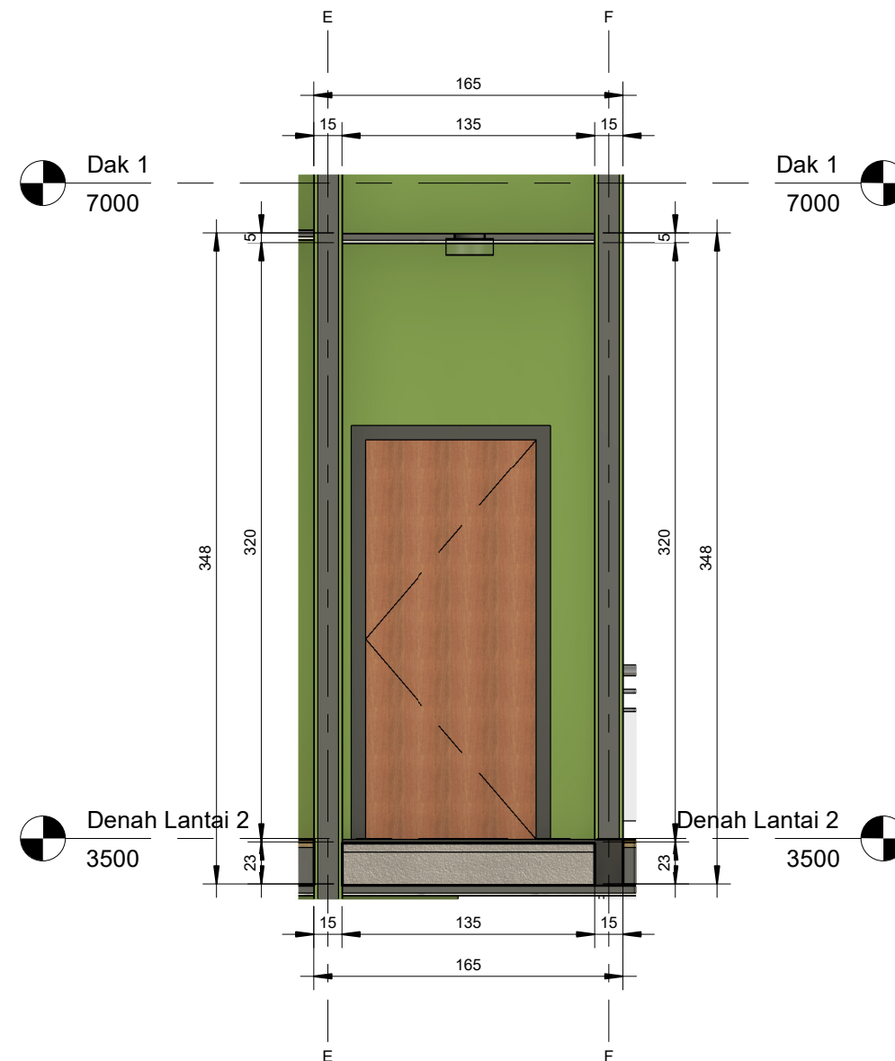
1 Toilet 2 - East 1 : 30
