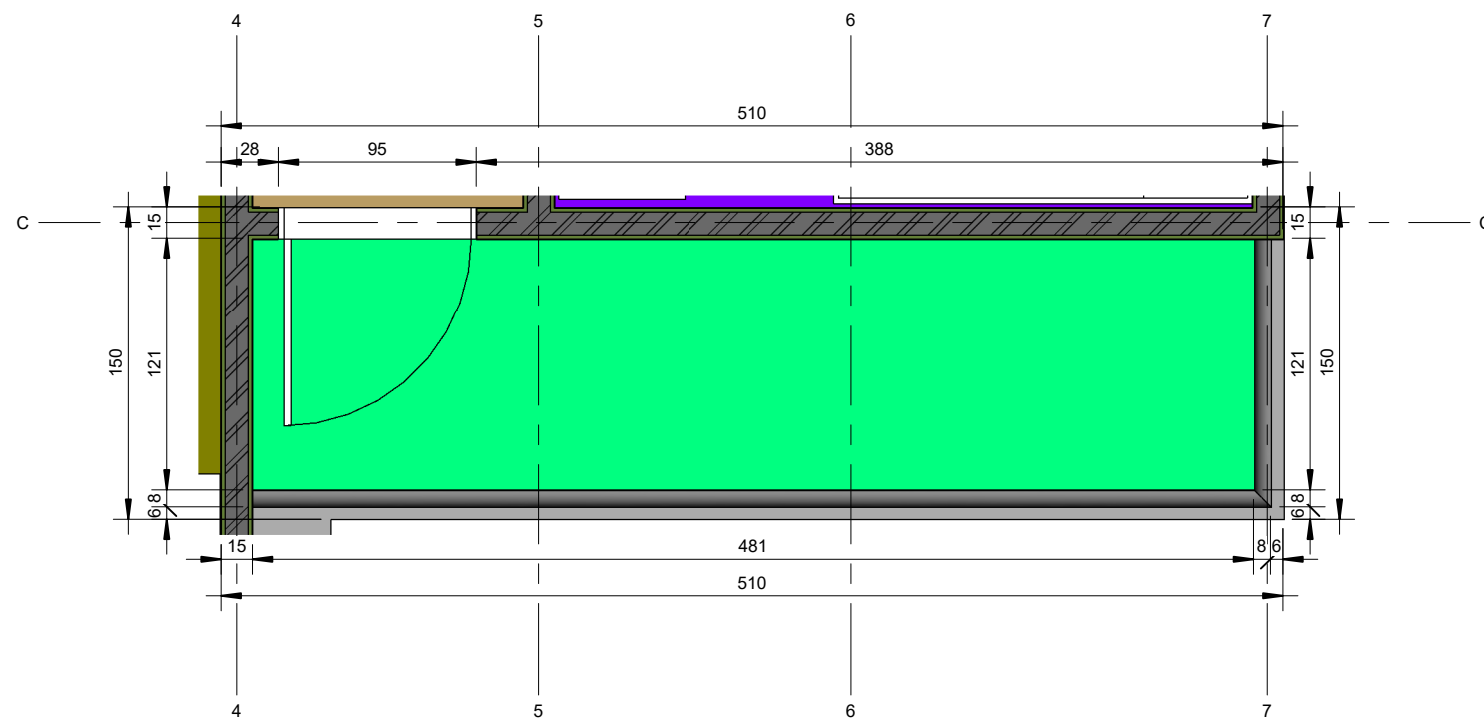
1 Denah Balkon 1 : 30
