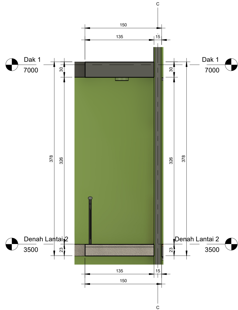
1 Balkon - East 1 : 30
