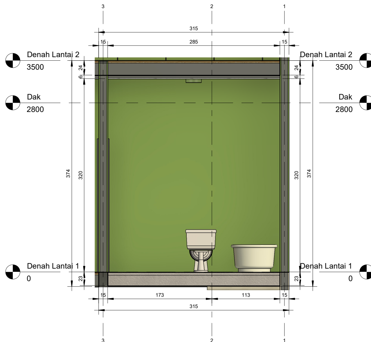
1 Toilet 1 - North 1 : 30
