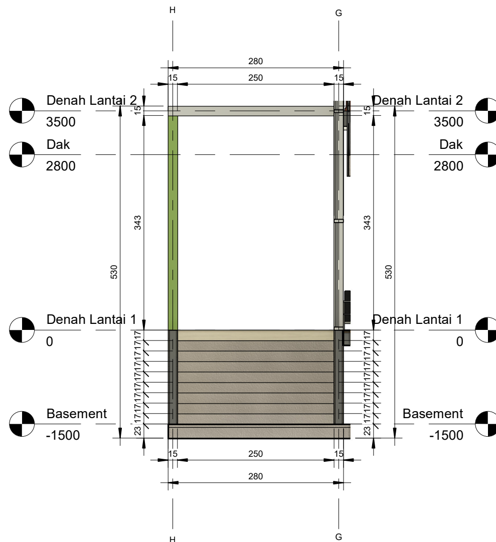
1 Teras - West 1 : 50
