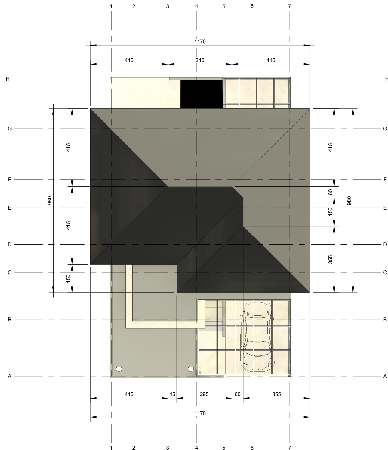
1 Site 1 : 100
