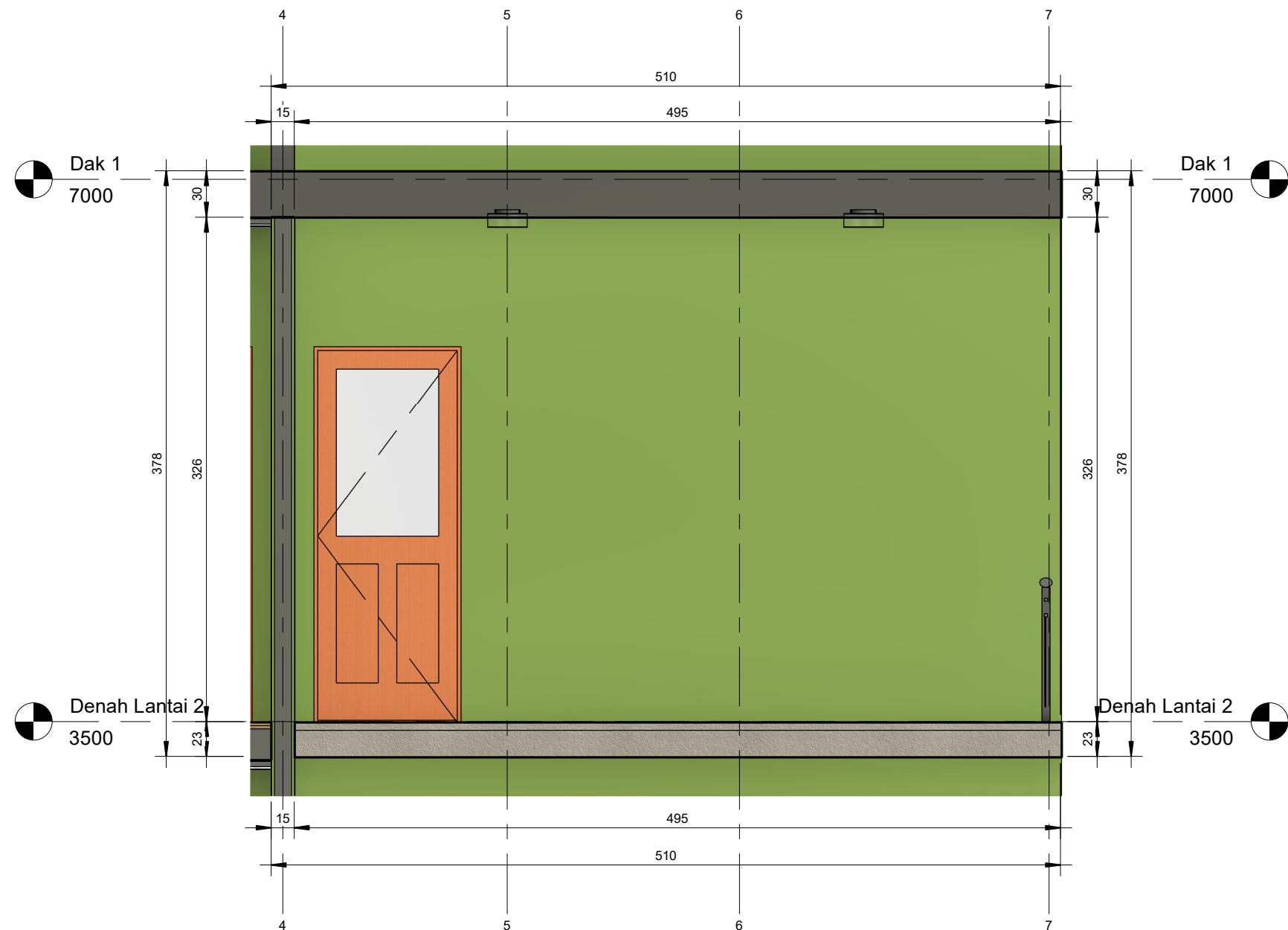
1 Balkon - South 1 : 30
