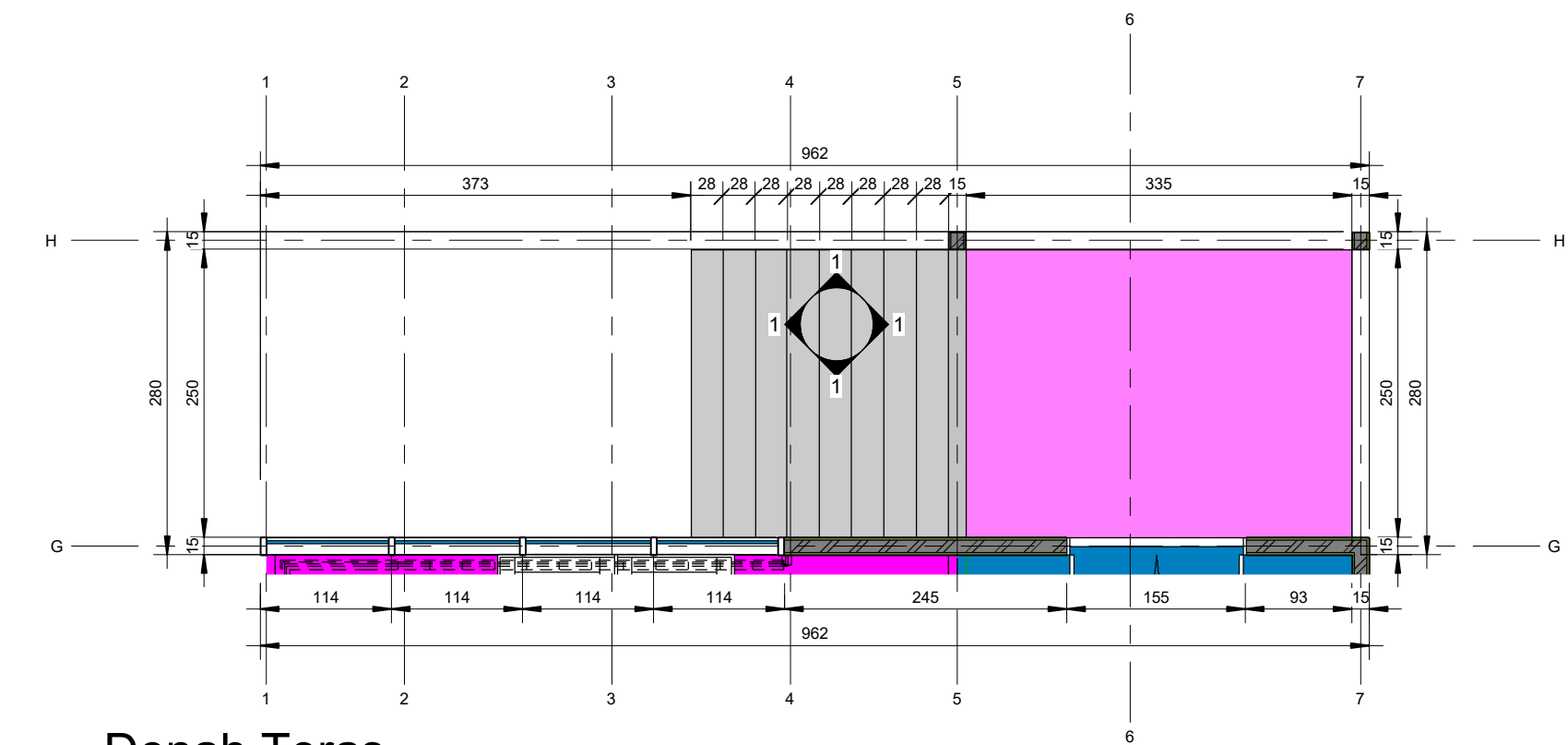
1 Denah Teras 1 : 50
