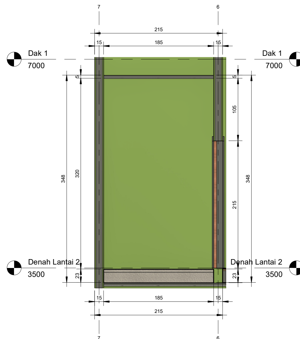
1 Toilet 2 - North 1 : 30
