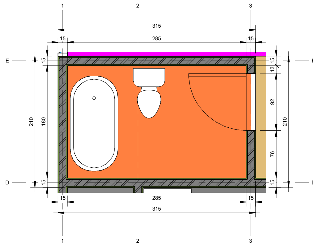
1 Denah Toilet 1 1 : 30
