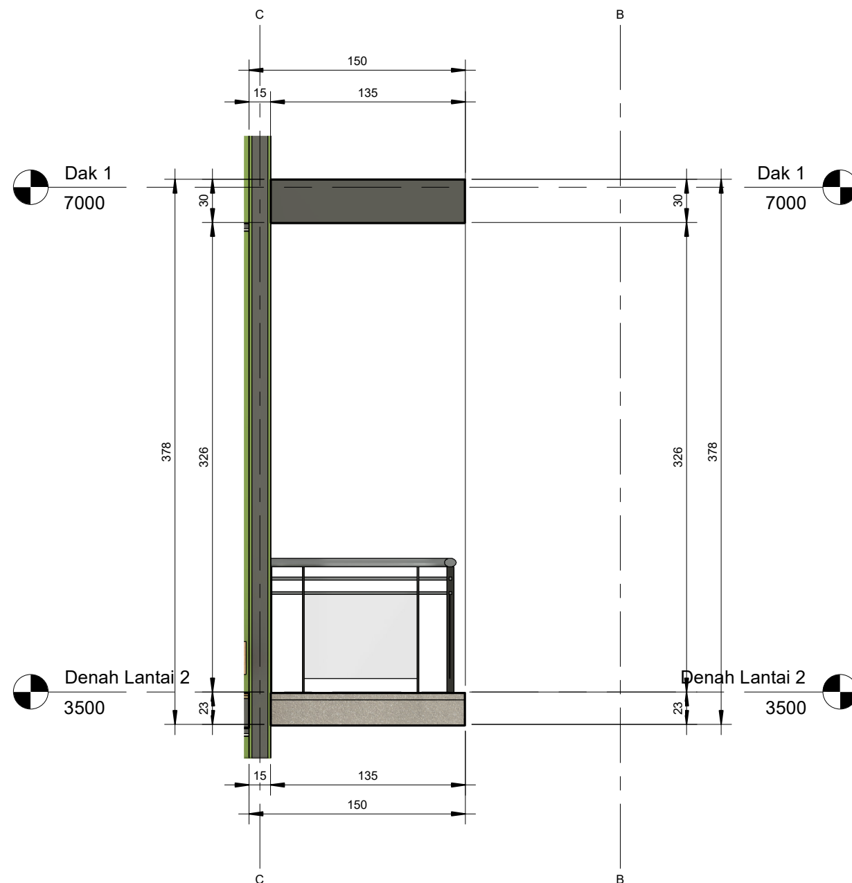
1 Balkon - West 1 : 30
