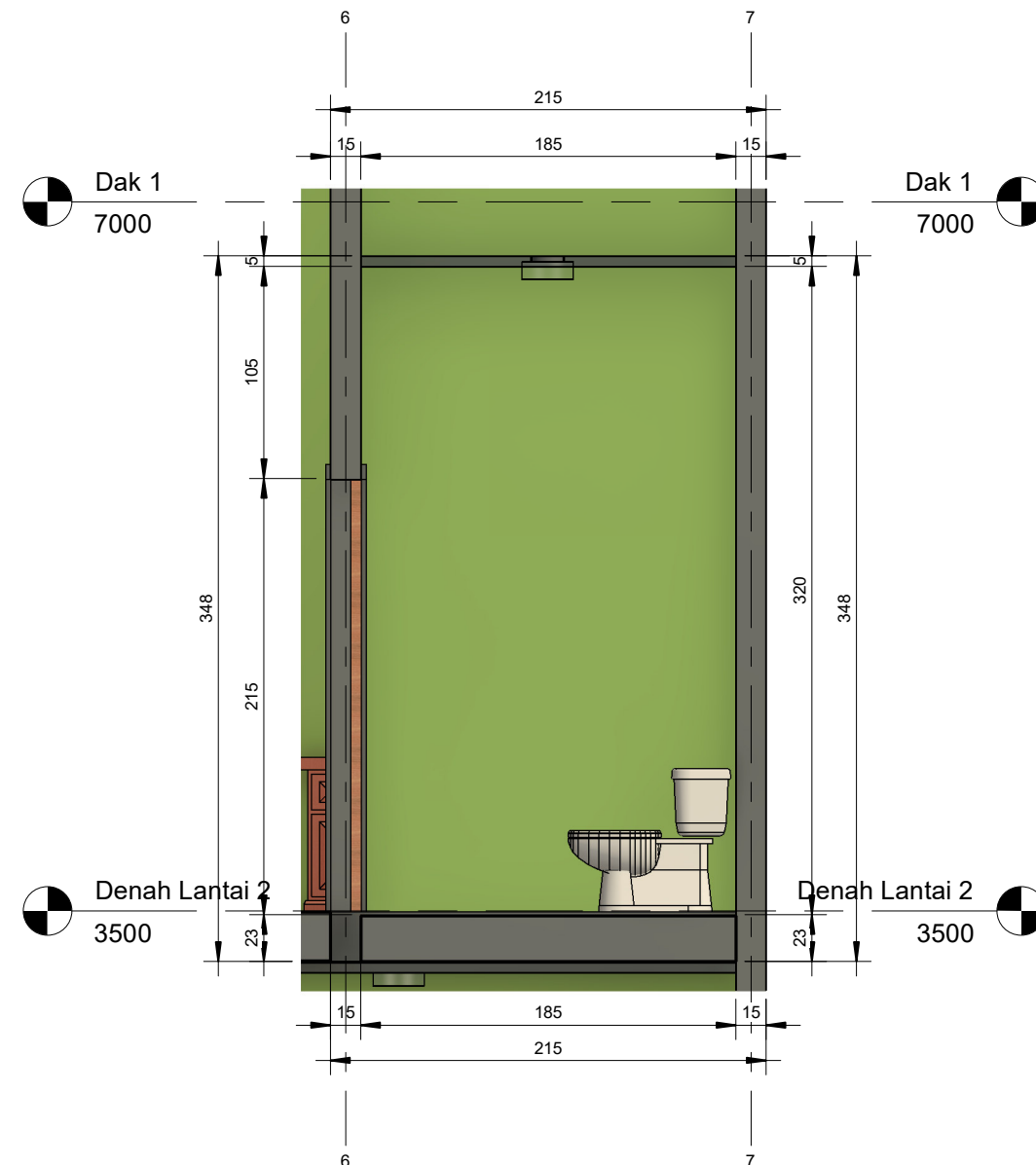
1 Toilet 2 - South 1 : 30
