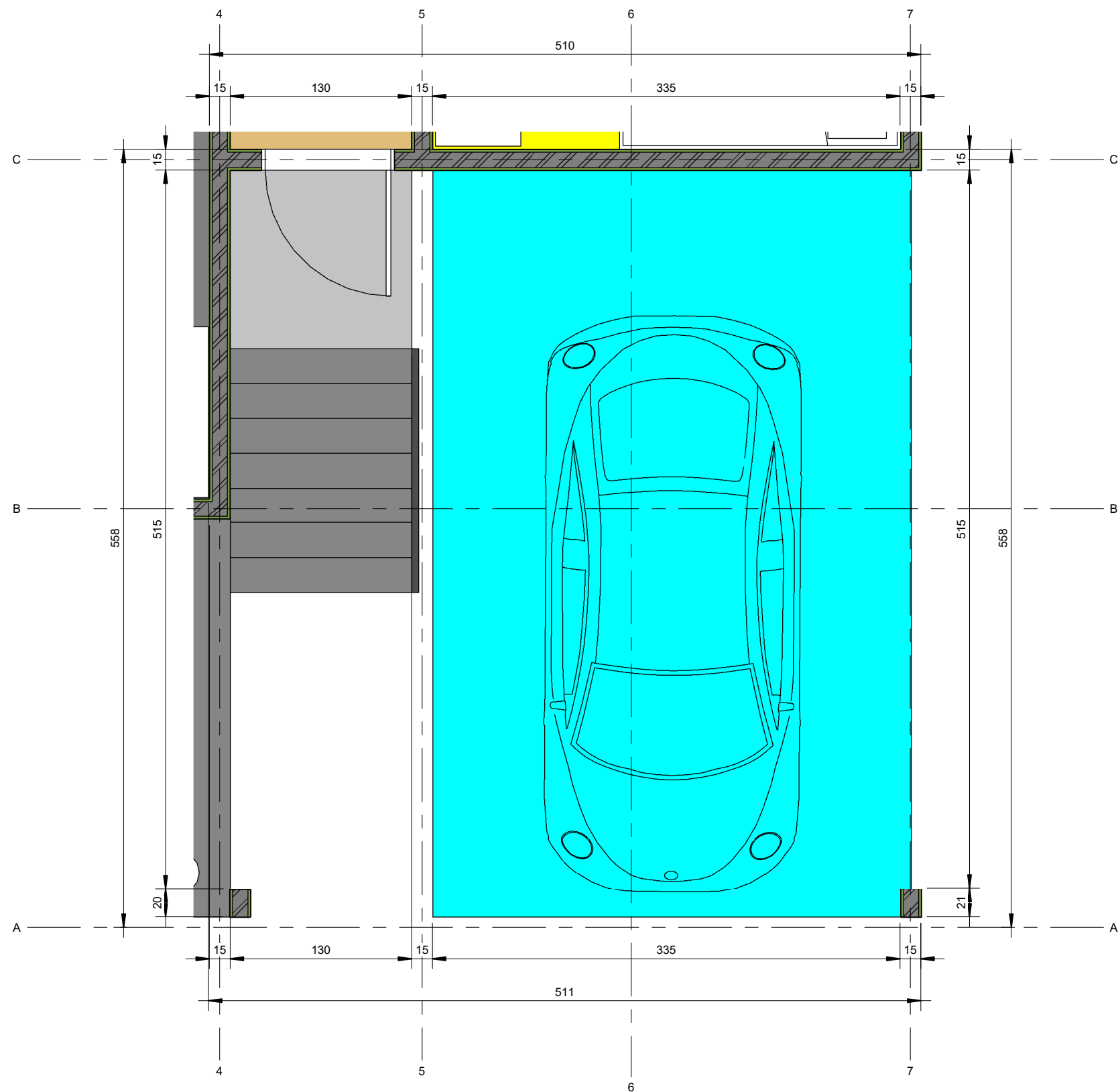
1 Denah Carport 1 : 30
