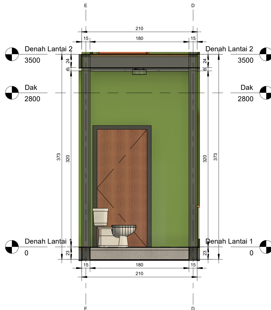
1 Toilet 1 - West 1 : 30
