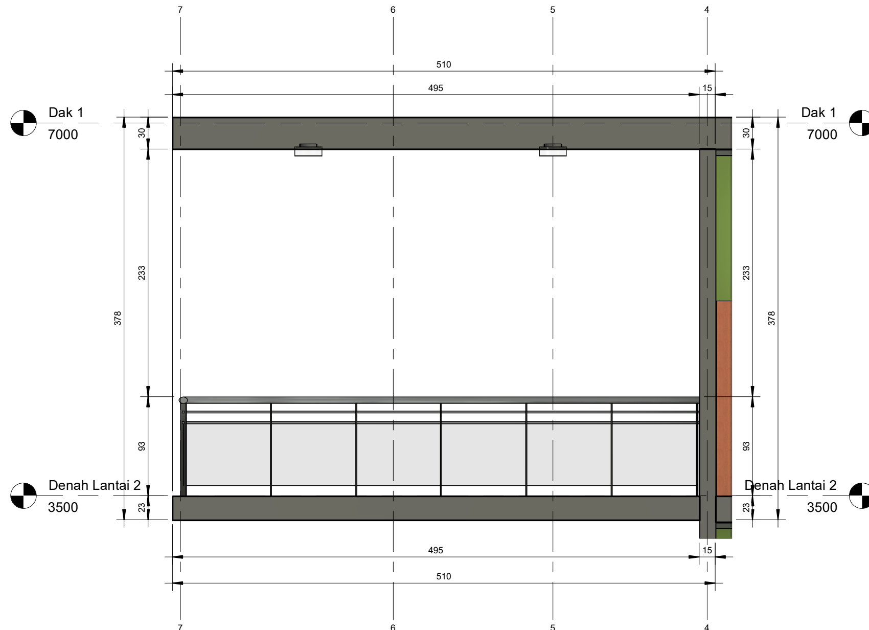
1 Balkon - North 1 : 30
