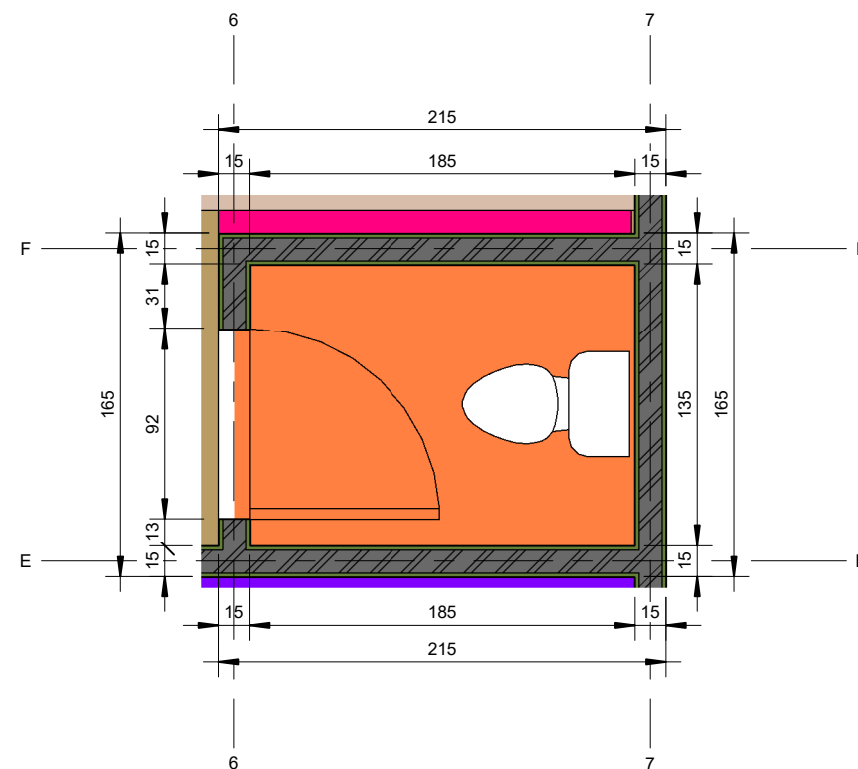
1 Denah Toilet 2 1 : 30
