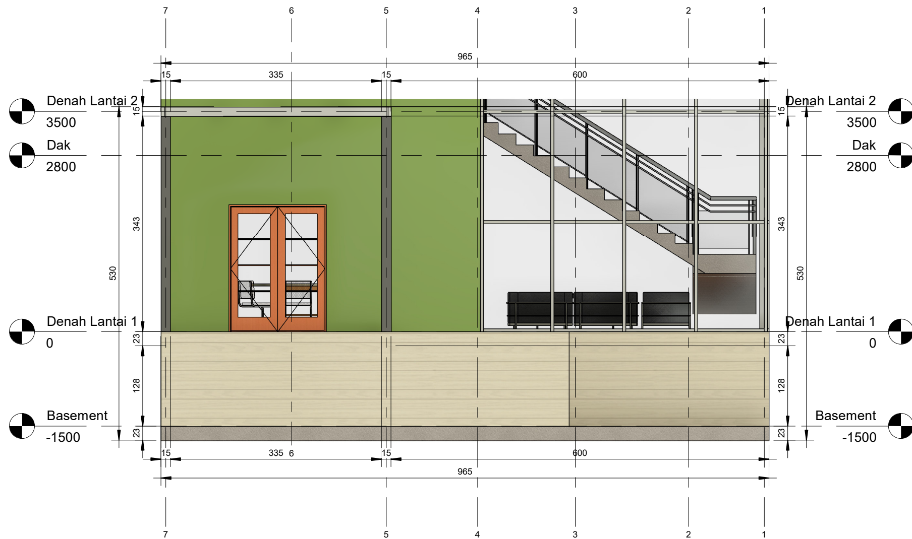
1 Teras - North 1 : 50
