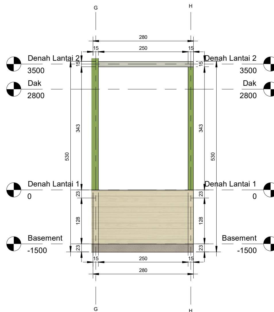
1 Teras - East 1 : 50
