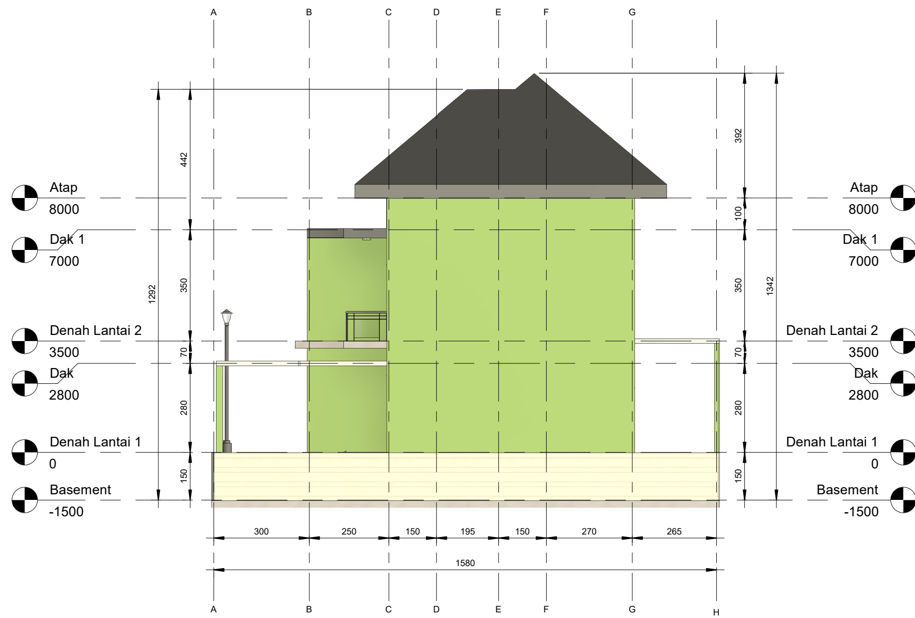
1 East 1 : 100
