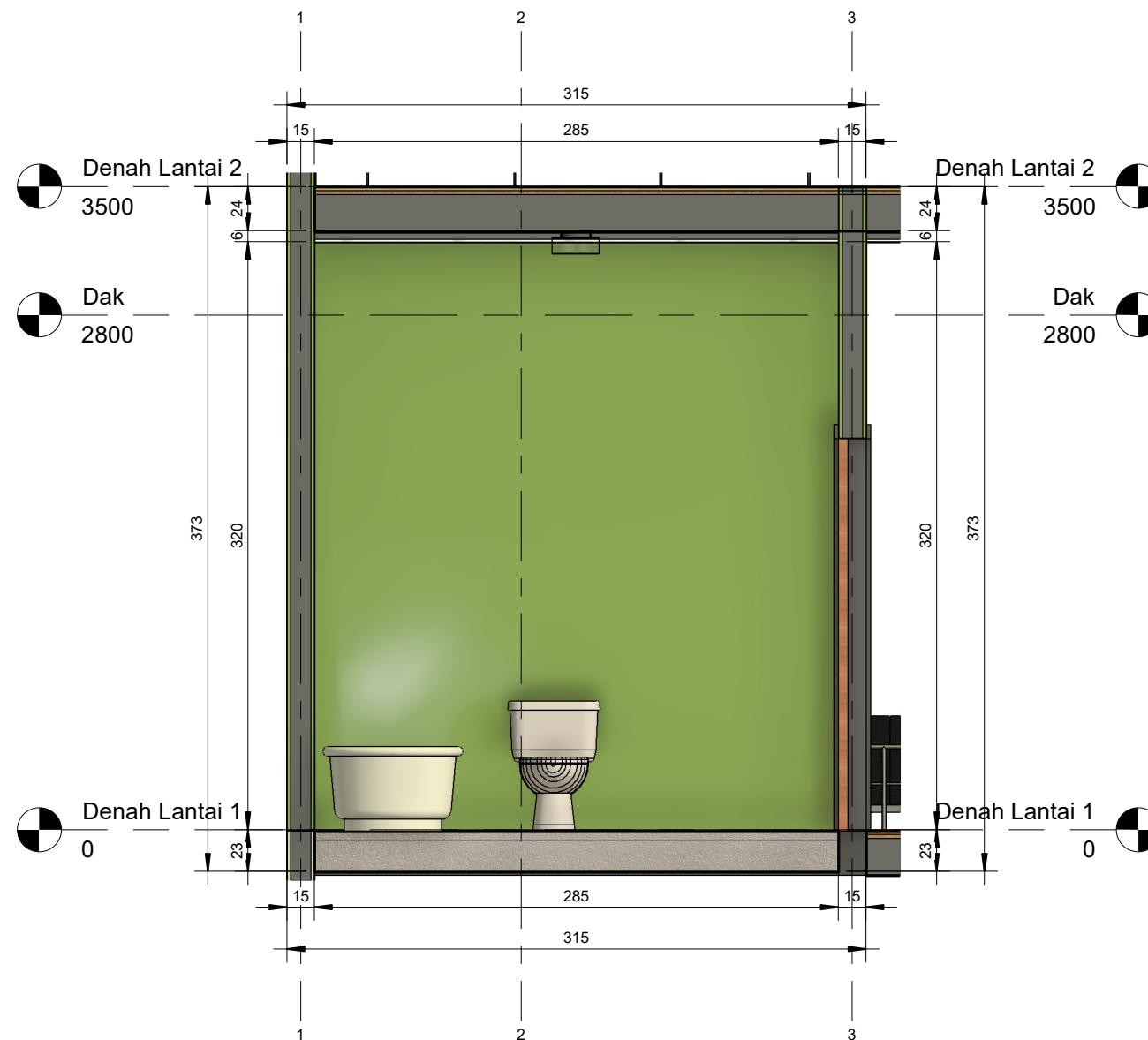
1 Toilet 1 - South 1 : 30
