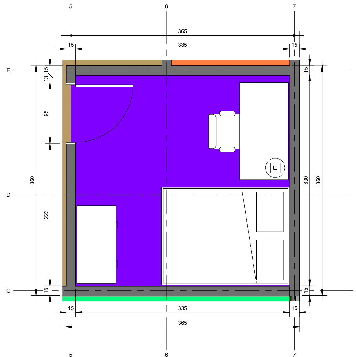
1 Denah Kamar 4 1 : 30
