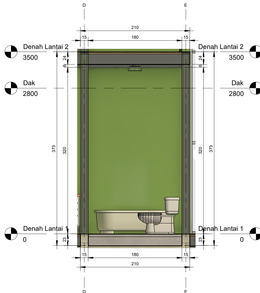
1 Toilet 1 - East 1 : 30
